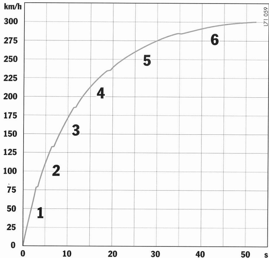
Diagramme d'accélération (Les valeurs sont communiquées pour un poids à vide selon la norme DIN et avec demi-charge, sans équipement supplémentaire.)
