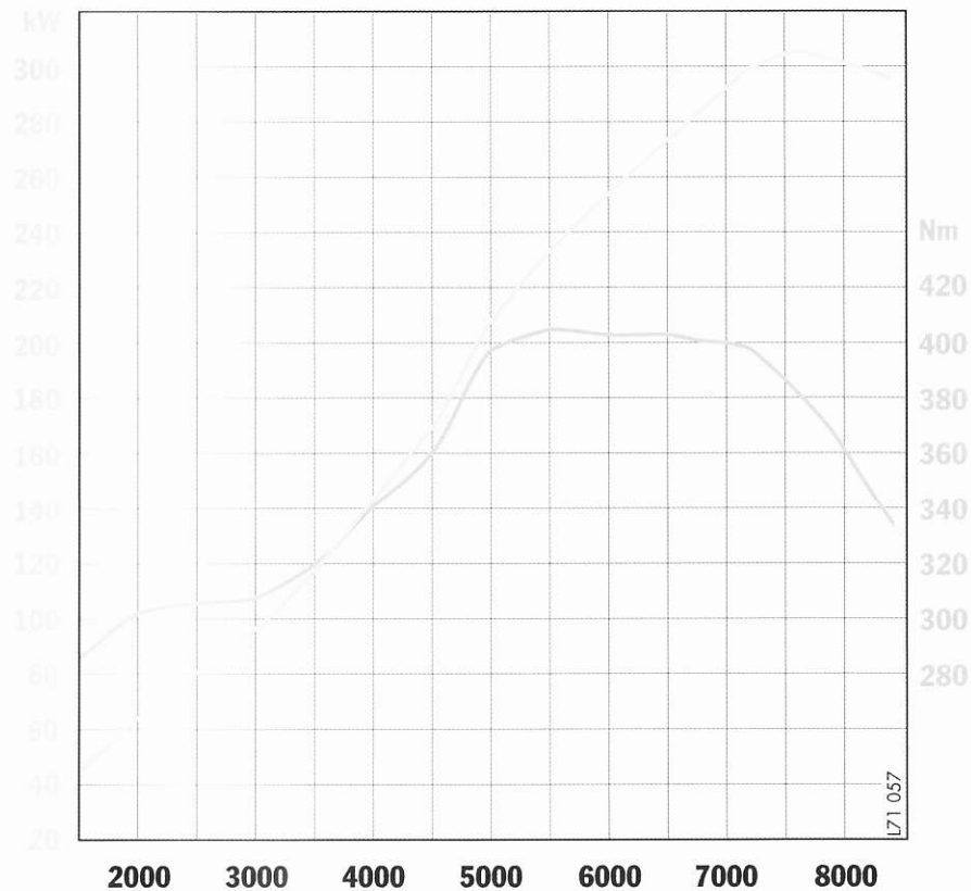
Diagramme moteur à pleine charge
