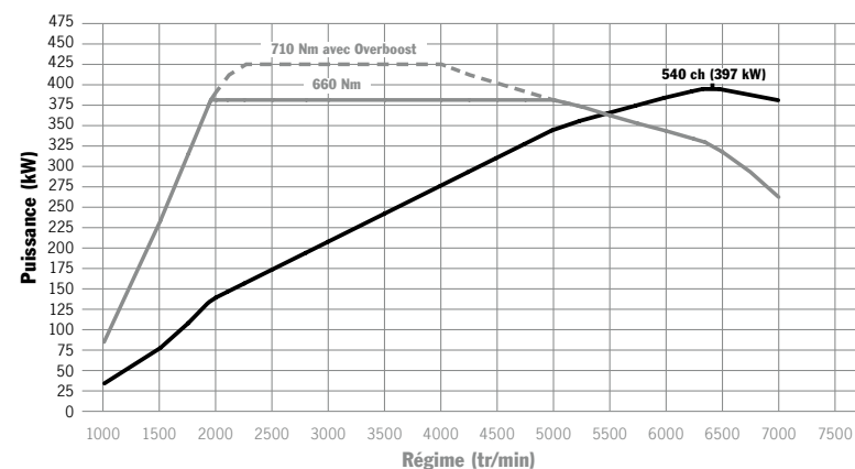
911 Turbo et 911 Turbo Cabriolet : 660 Nm entre 1 950 et 5 000 tr/min (avec Overboost : 710 Nm entre 2 250 et 4 000 tr/min), 540 ch (397 kW) à 6 400 tr/min
