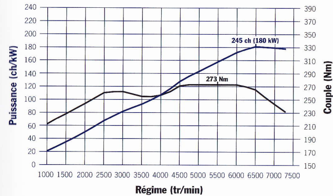
Boxster : 273 Nm entre 4 600 et 6 000 tr/min, 245 ch (180 kW) à 6 500 tr/min
